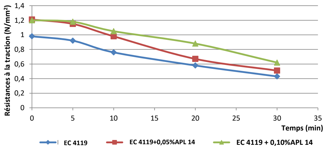
Effet du Pentamix APL 14 sur les résistances à la traction des un ciment-colle formulée avec notre cellulose modifiée Penta EC 4119
