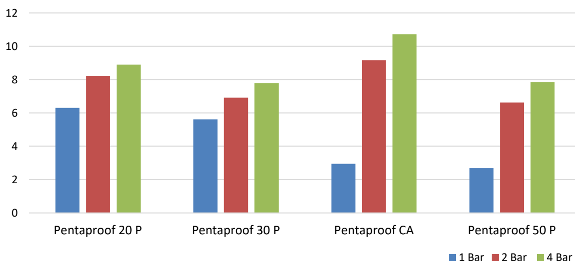
Absorption d'eau des produits Pentaproof à différentes pressions d'eau (dosage 1,0% sur le ciment)
